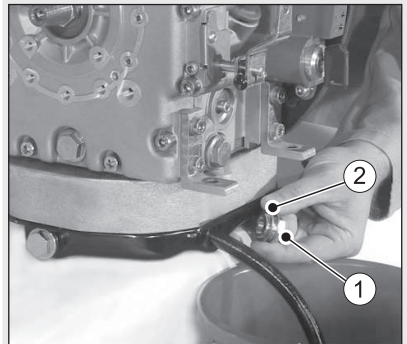
Met oliecarter
