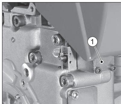
1 Brandstofafsluitklep
