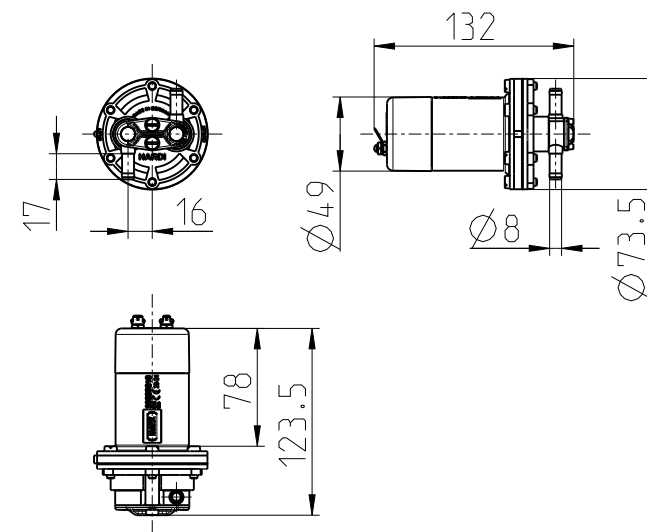
Kraftstoffförderpumpe FUEL DELIVERY PUMP
