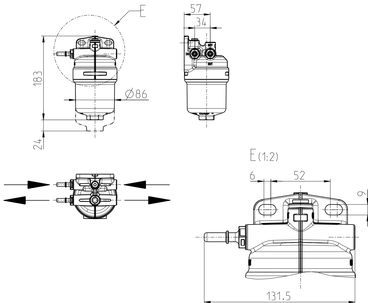
Kraftstoffhauptfilter FUEL MAIN-FILTER
