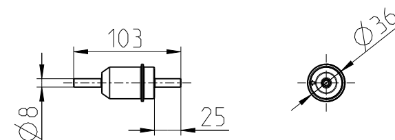
Kraftstoffvorfilter FUEL PRE-FILTER
