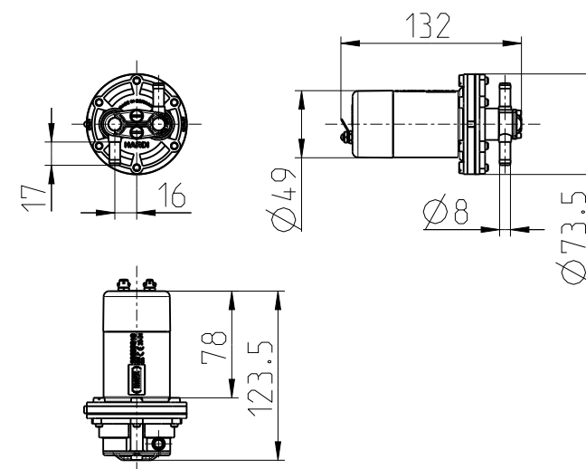
Kraftstoffförderpumpe FUEL DELIVERY PUMP
