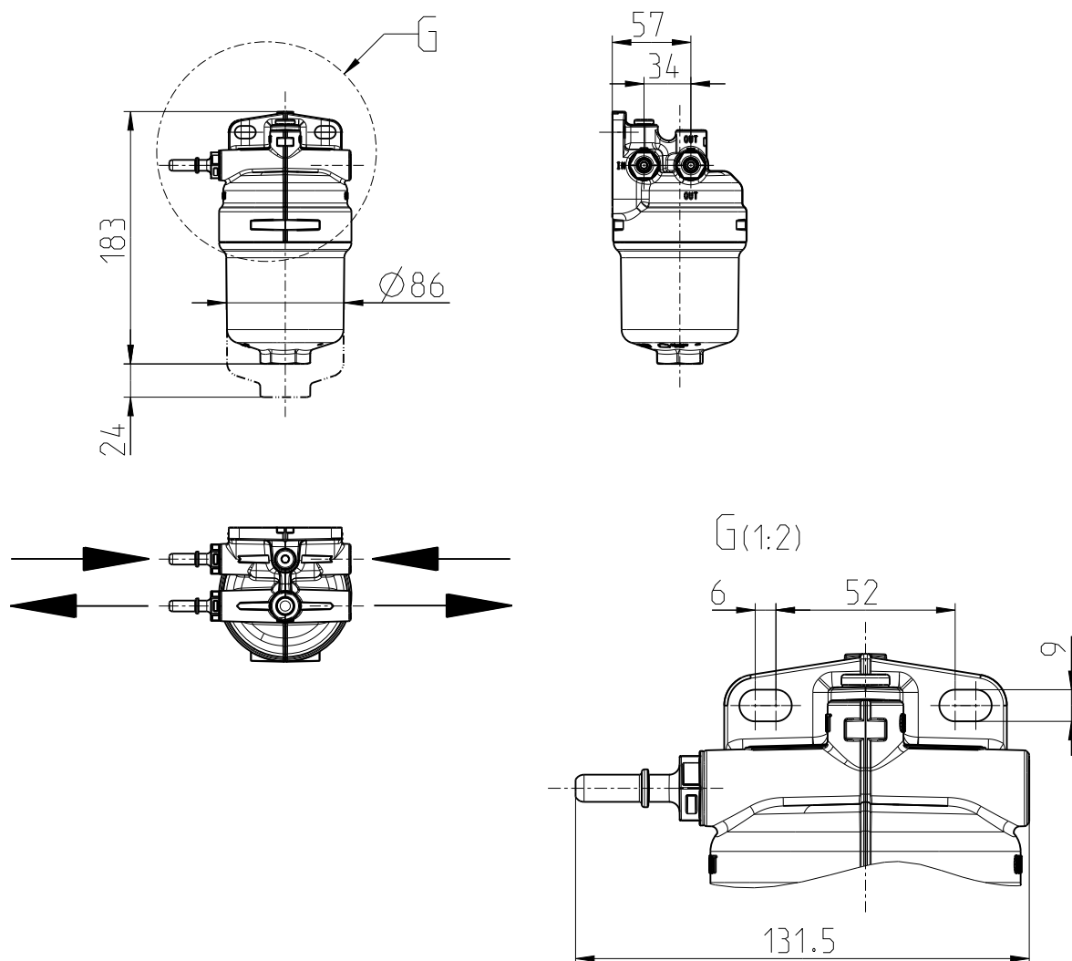
Kraftstoffhauptfilter FUEL MAIN-FILTER
