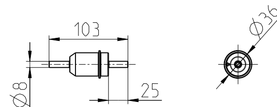
Kraftstoffvorfilter FUEL PRE-FILTER
