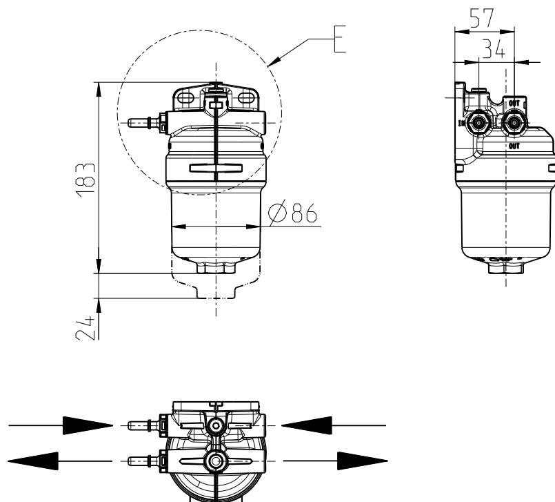
Kraftstoffhauptfilter FUEL MAIN-FILTER
