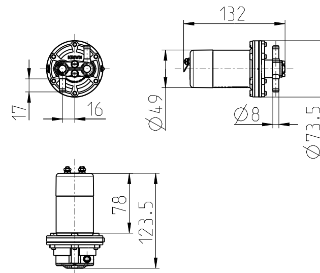
Kraftstoffförderpumpe FUEL DELIVERY PUMP
