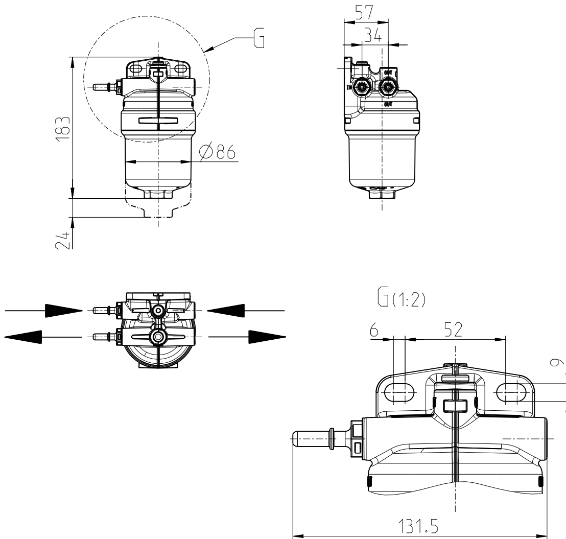
Kraftstoffhauptfilter FUEL MAIN-FILTER
