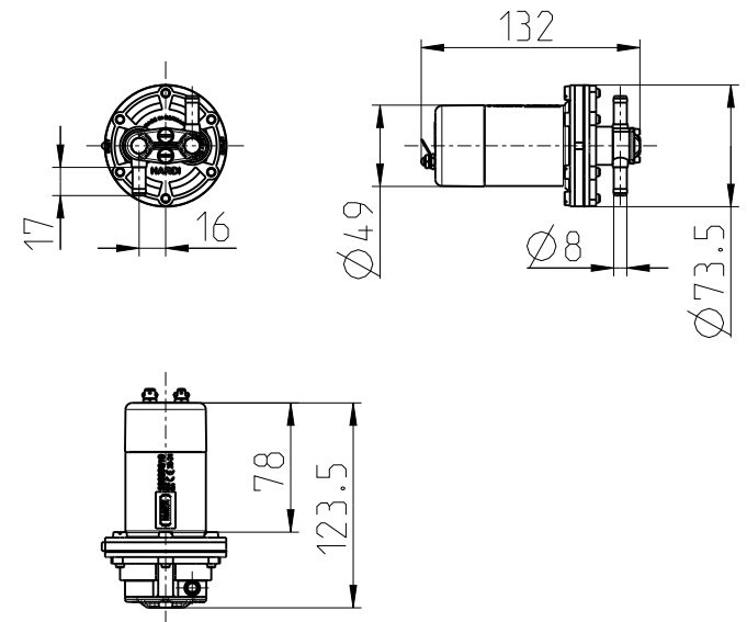
Kraftstoffförderpumpe FUEL DELIVERY PUMP
